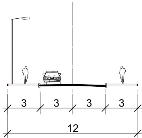
Поперечний профіль 1-1
