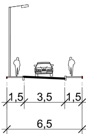
Поперечний профіль 2-2
