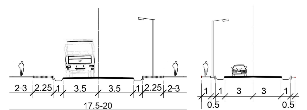
Профіль 1-1
